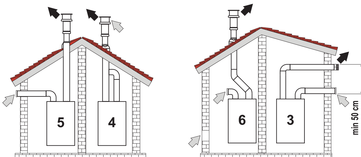
fig. 19 - Ejemplos de conexión con tubos separados (⇐ = aire / ➡ = humos)
