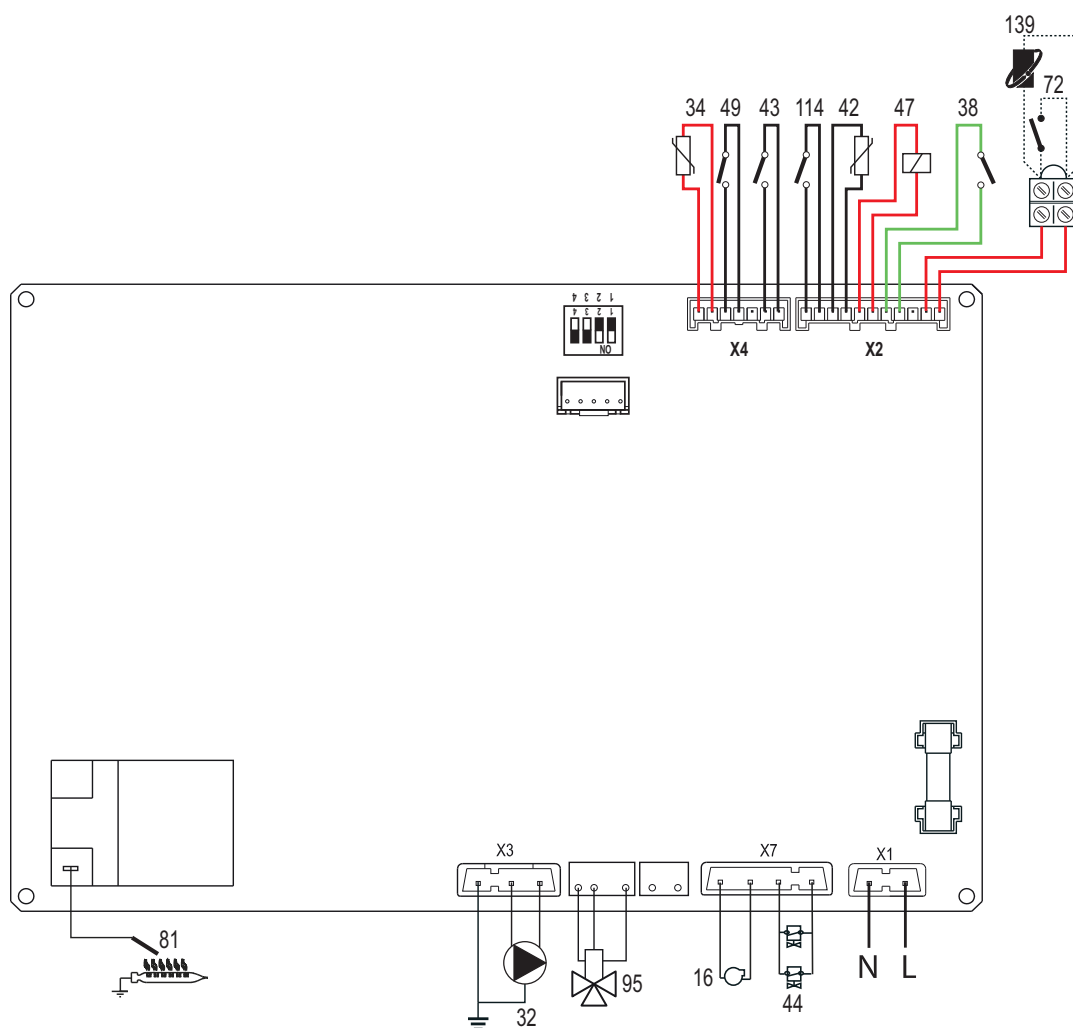
fig. 54 - Esquema eléctrico
