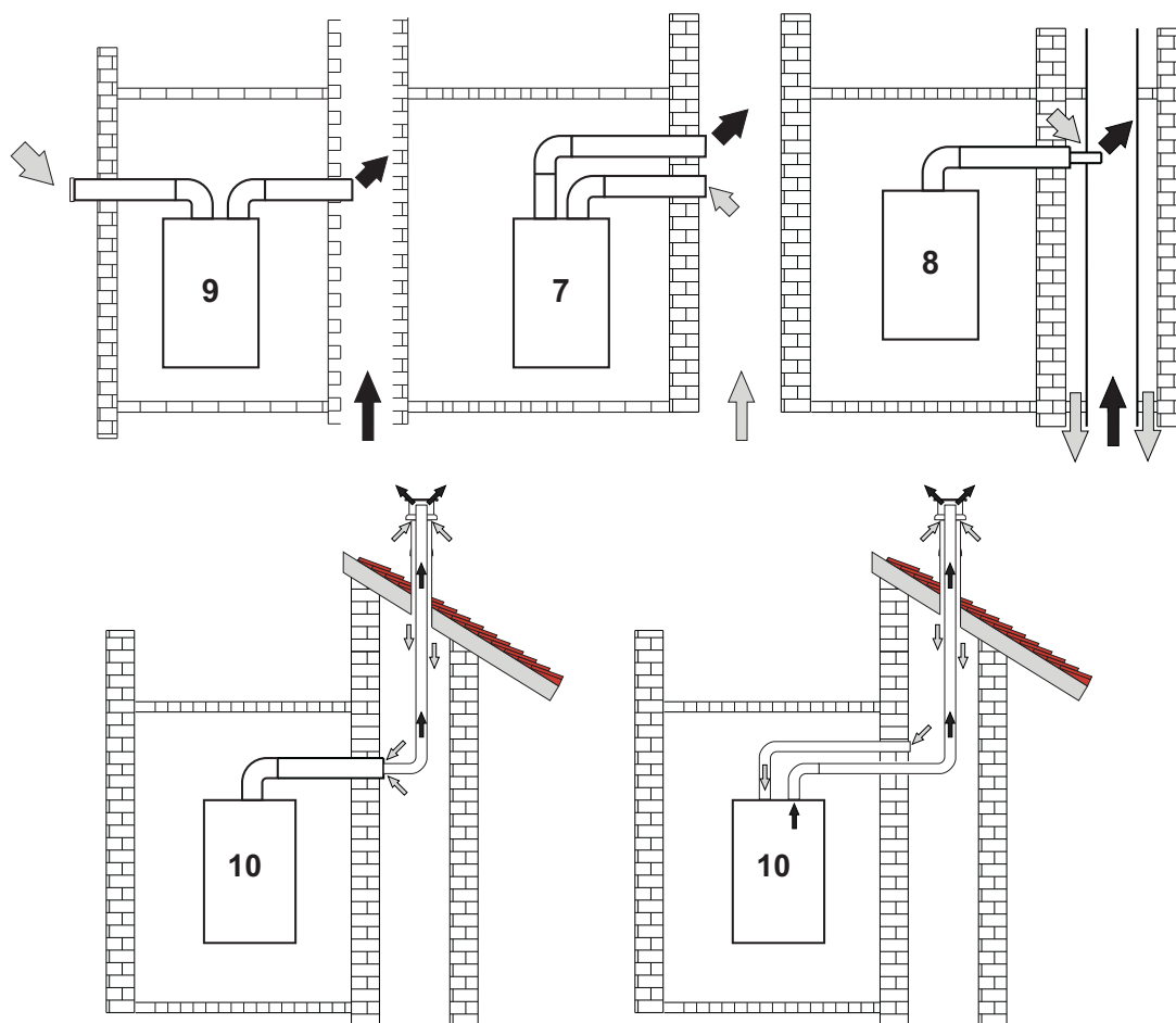
fig. 25 - Ejemplos de conexión a chimeneas (⇐ = aire / ⇨ = humos)
