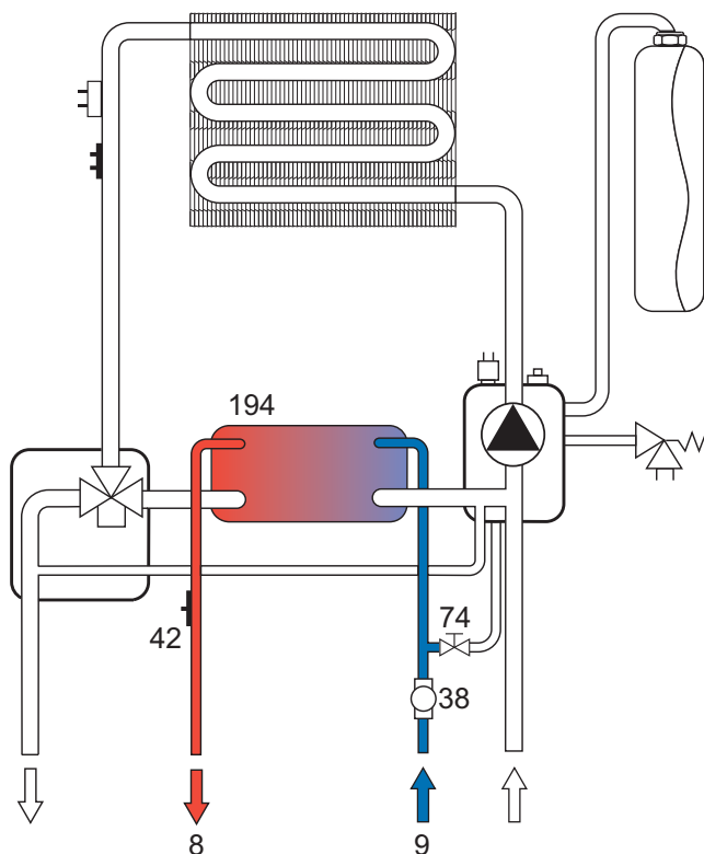
fig. 53 Circuito sanitario
