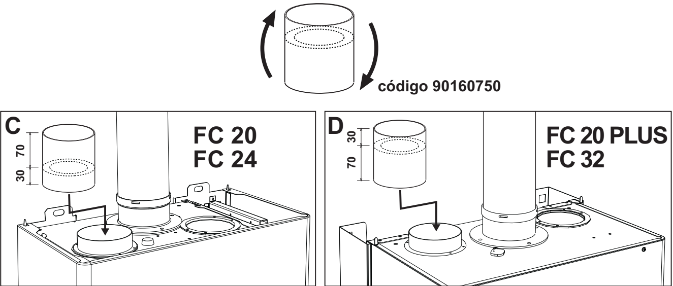
fig. 55 - Inserción del manguito
