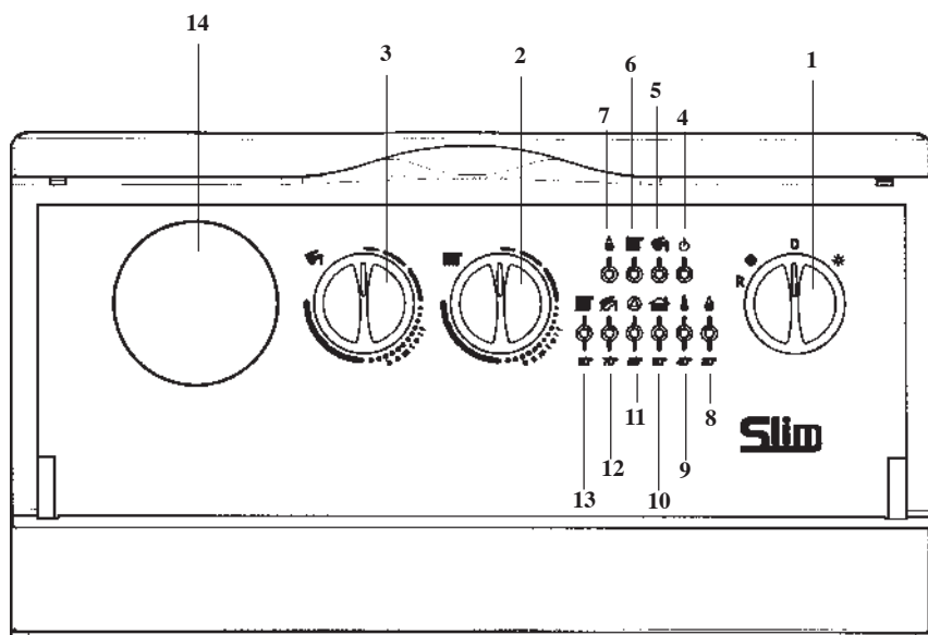
Figura 1: cruscotto caldaia
